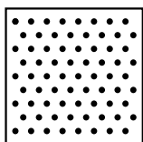
Padrão (Ø): Microperfurado Diâmetro furo: Ø 2 mm Área aberta: 15%
